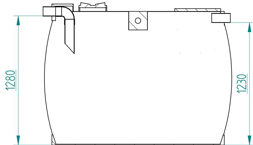
COUPE A-A
