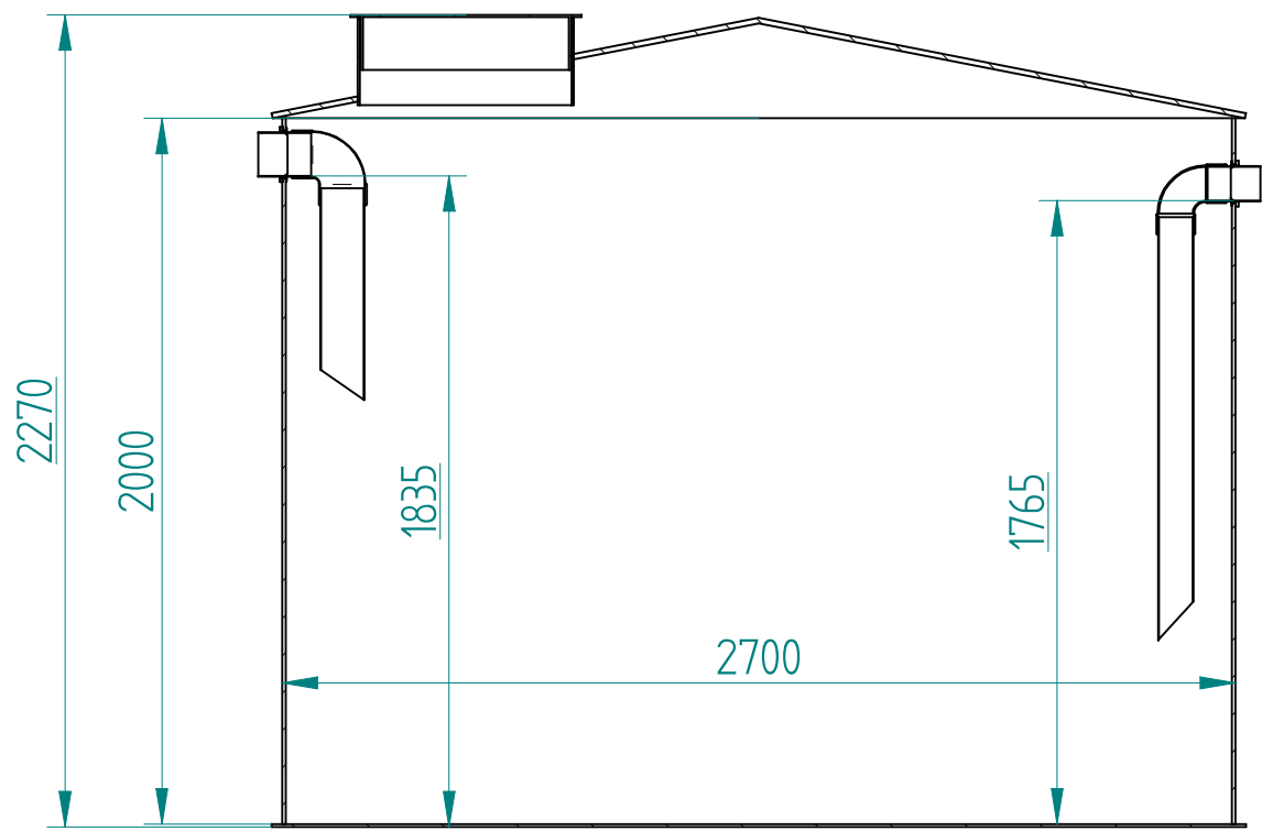
COUPE A-A
