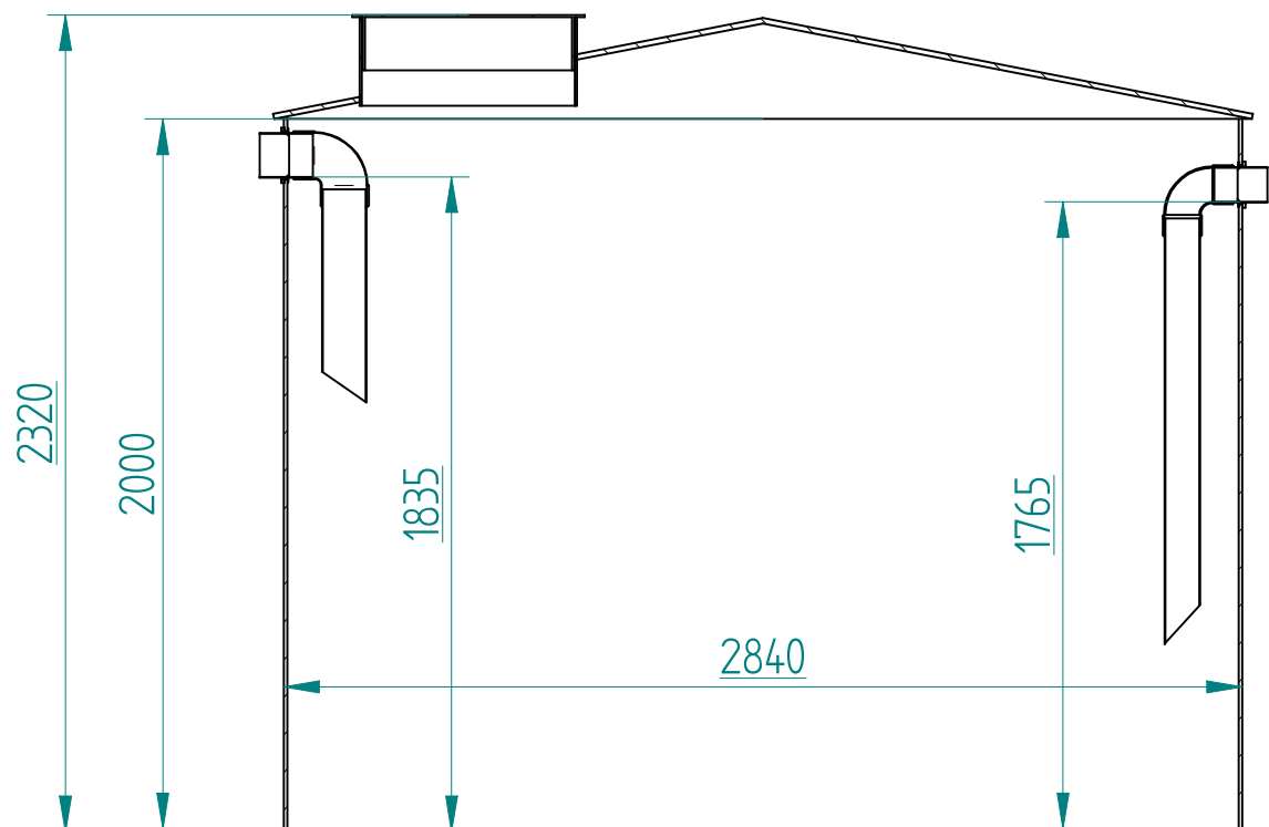
COUPE A-A
