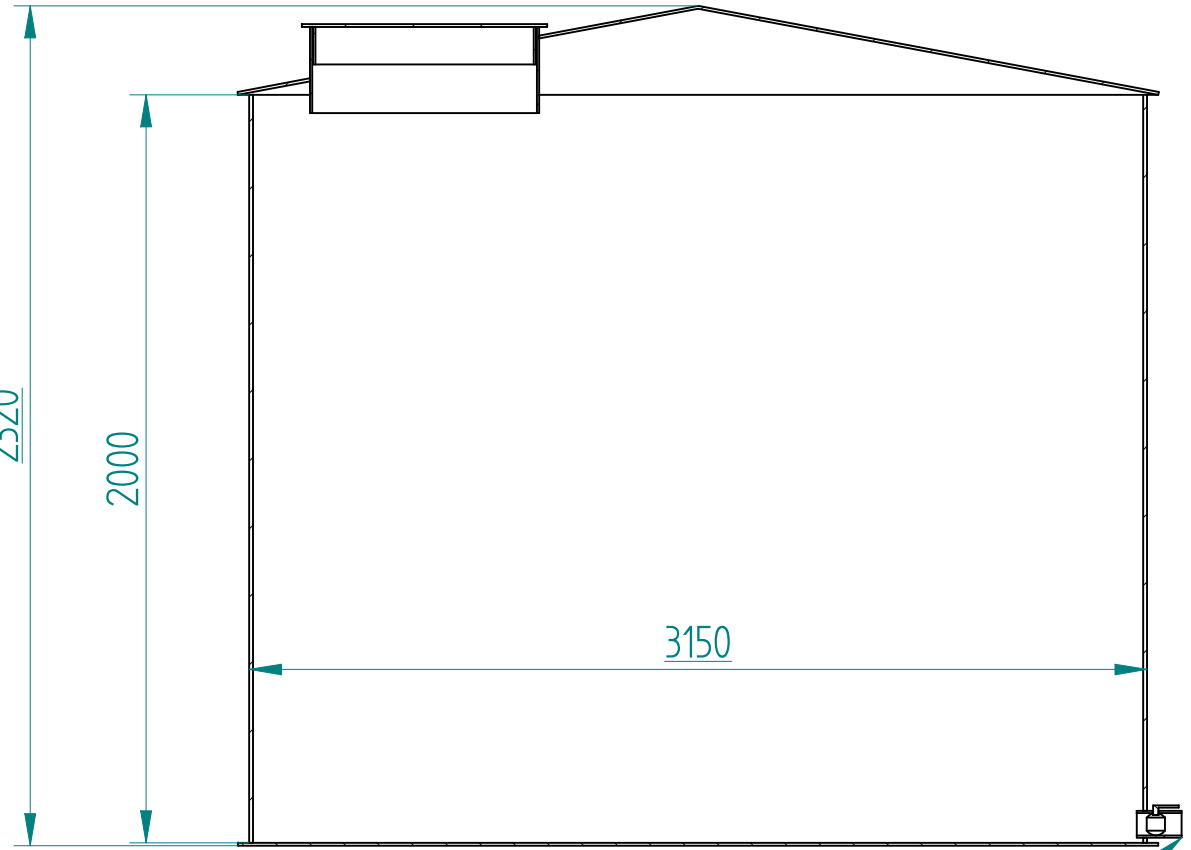
COUPE A-A
