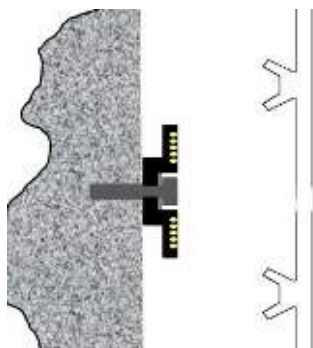
Figure 11. Rondelle PE
