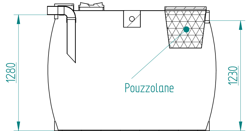
COUPE A-A
